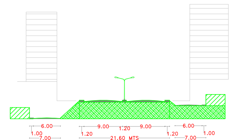
CORTE ESQUEMATICO A-A'
