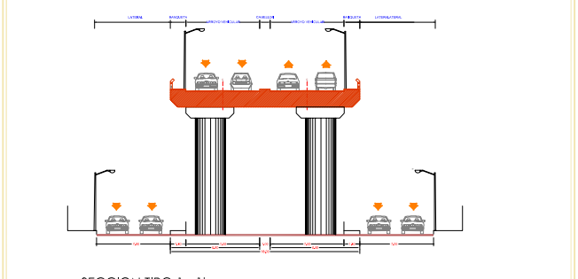
SECCION TIPO 1 - 1' PROYECTO ESC: 1/4 NOTA: LA REPRESENTACION DE ESTE PLAN ES GENERAL Y SUJETA A CAMBIOS.
