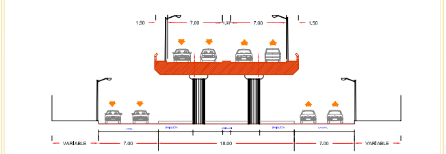
SECCION TIPO 1 - 1' PROYECTO ESC: SIN
